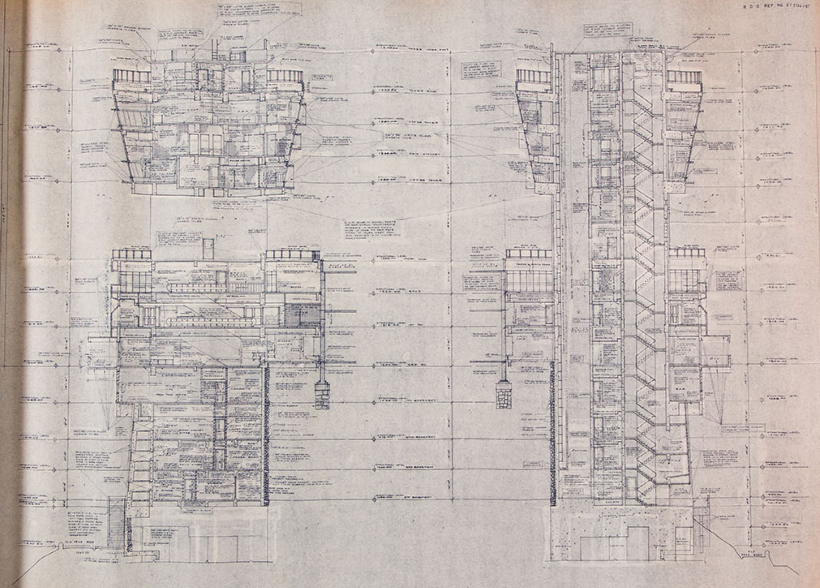
SECTION A-A
